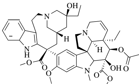
53 vinblastine
